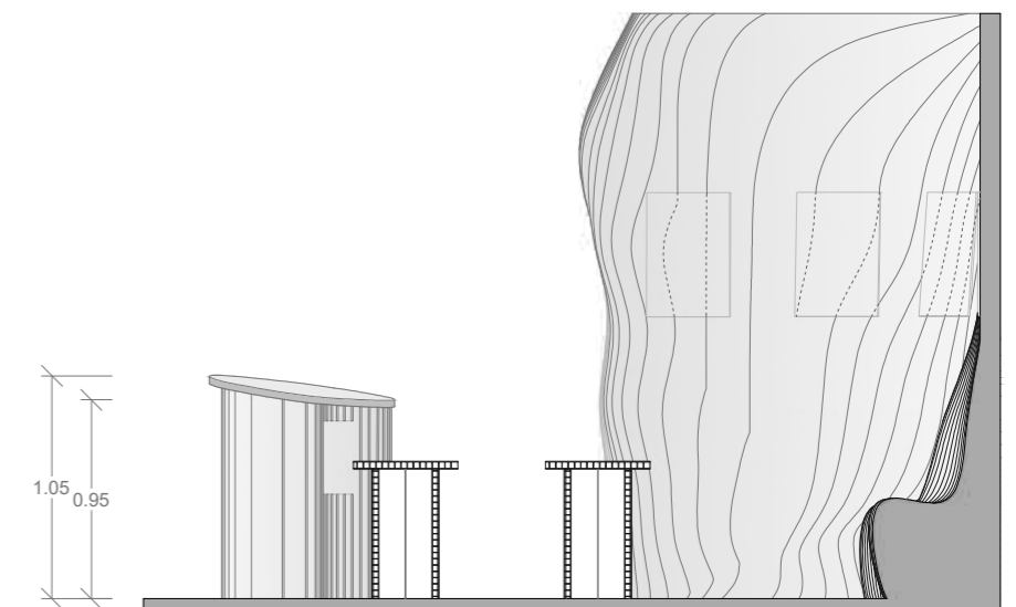
Sección transversal
